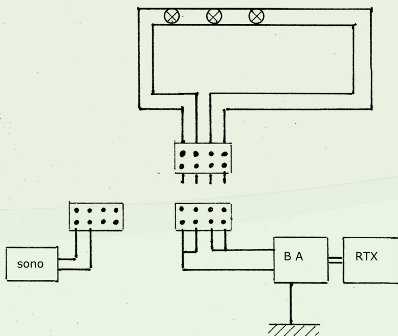
fig 4 antenne boucle
